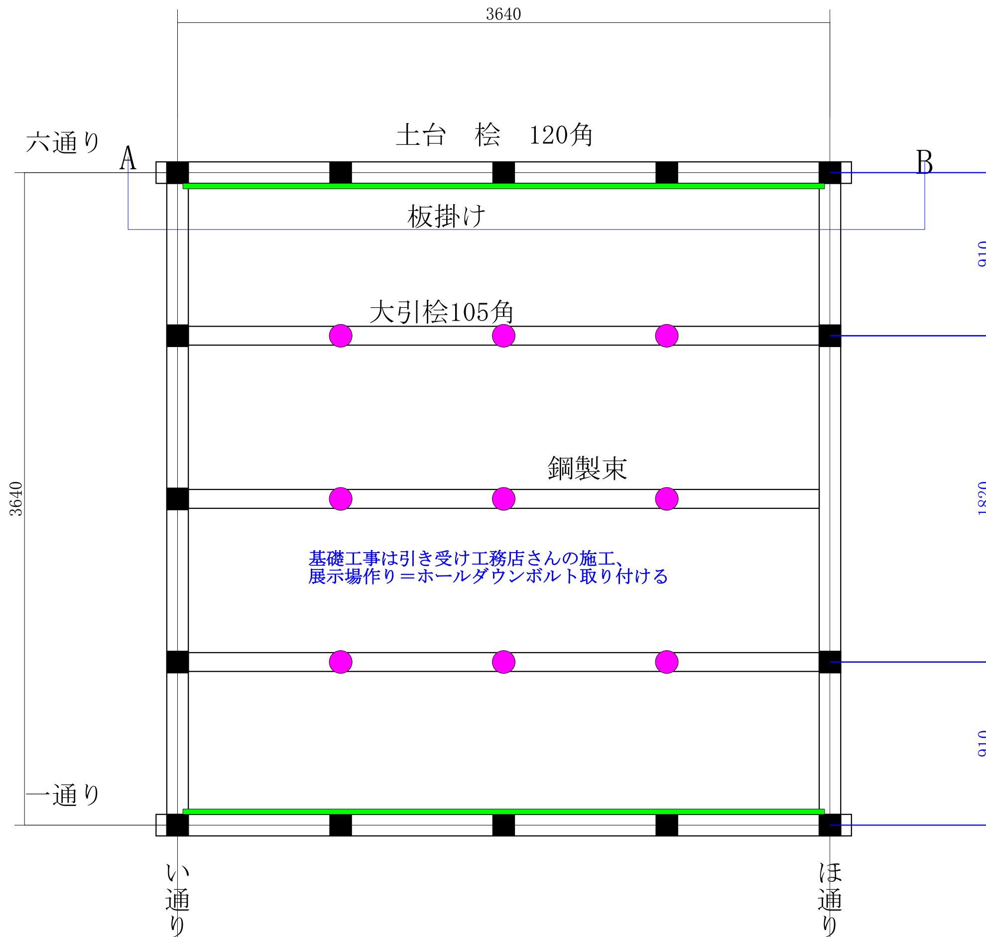
平面図＋柱伏図＋床伏図
