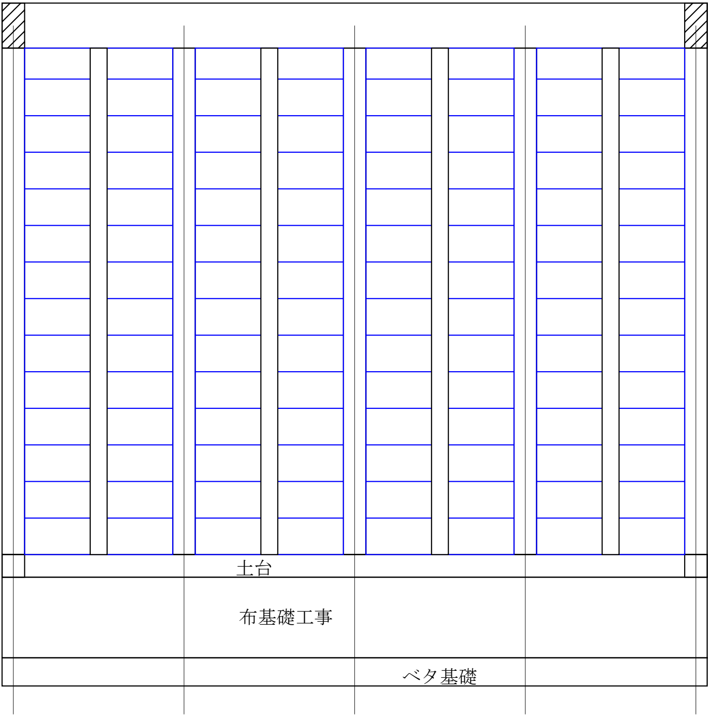
一通り字裏 展開図 土壁パネル
